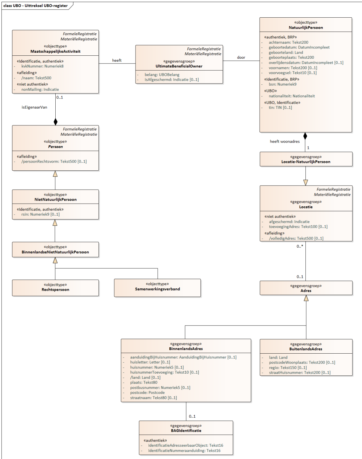
Figuur 3: Gegevensmodel productgegevens
